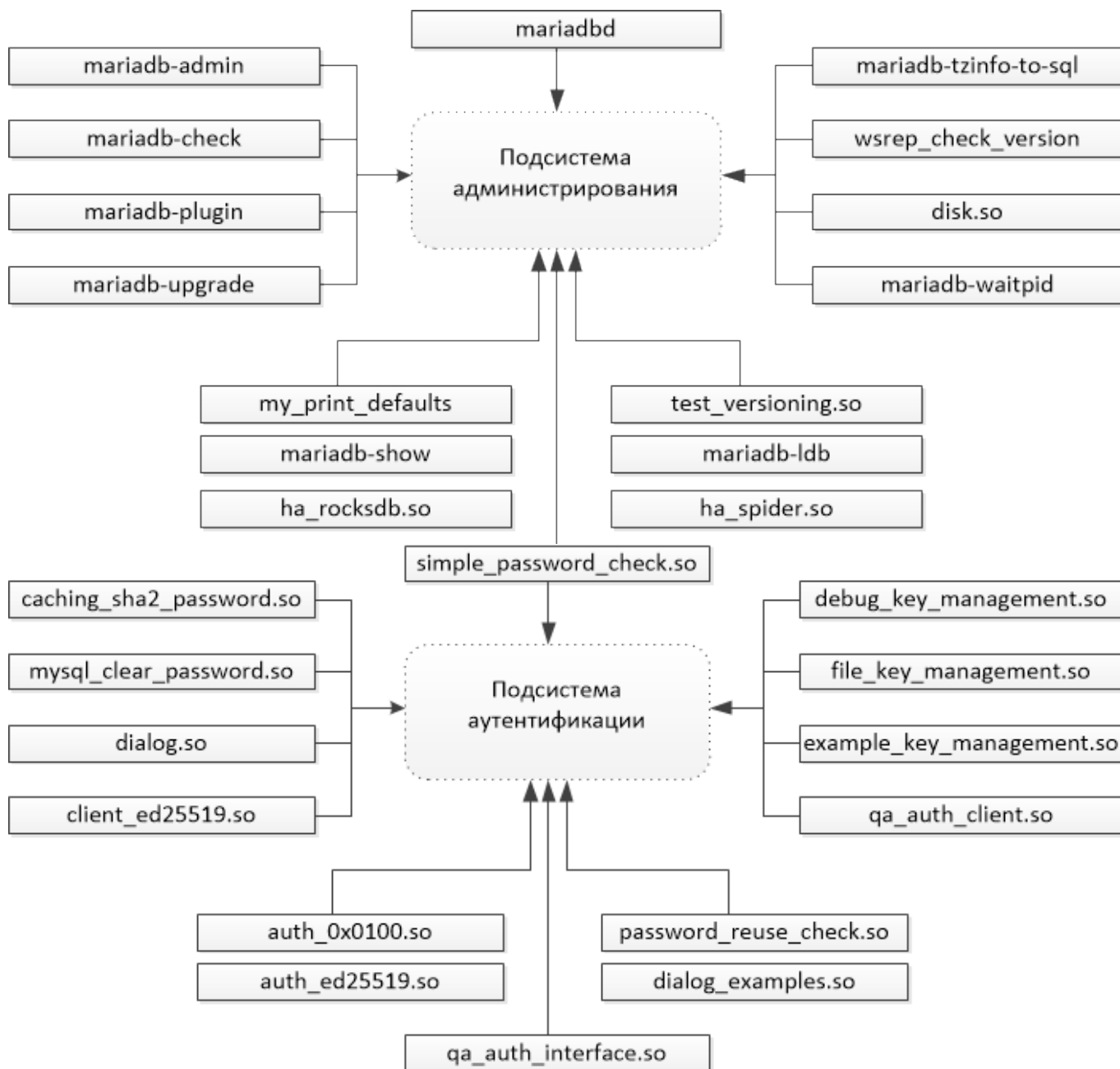
Рис.1 Структура подсистемы Администрирования в СУБД «КАТРАПС»
