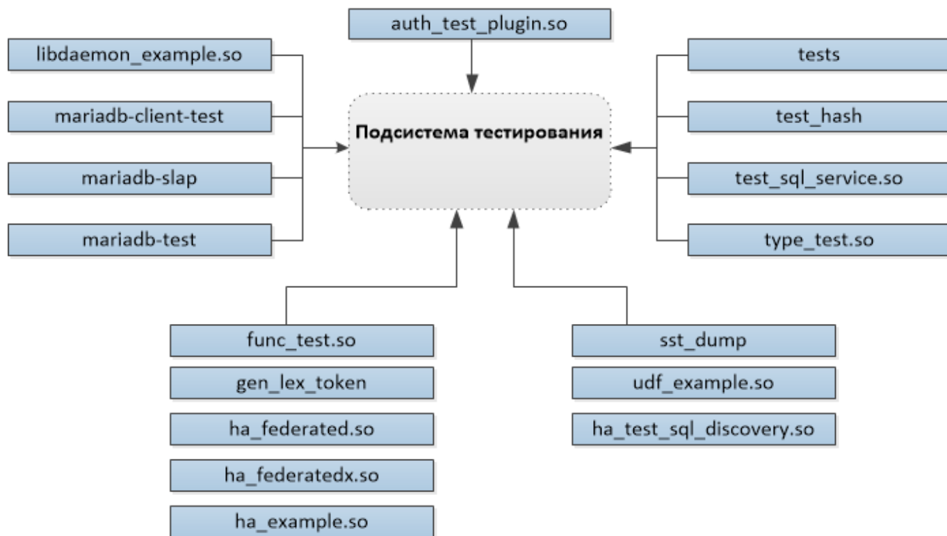
Рис.5 Структура подсистемы Тестирования в СУБД «КАТРАПС»
