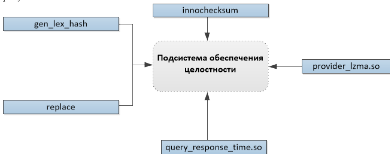
Рис.2 Структура подсистемы Обеспечения целостности в СУБД «КАТРАПС»
