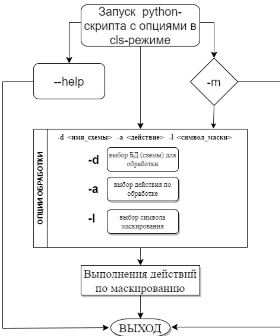
Рис.7 Функционирование модуля маскирования СУБД «КАТРАПС».
