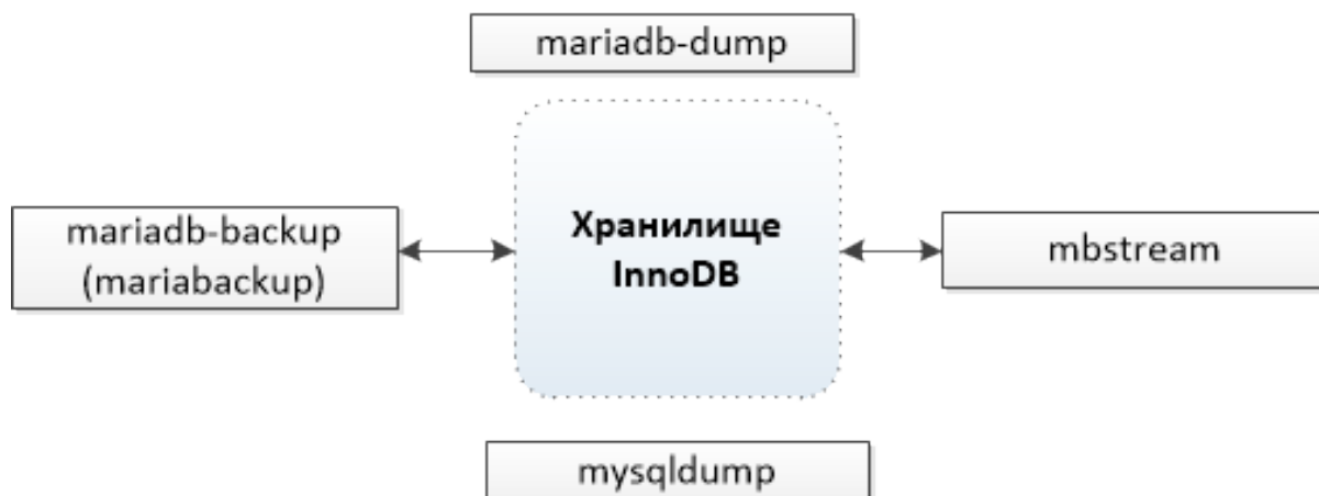
Рис.4 Структура подсистемы Резервного копирования и репликации в СУБД «КАТРАПС»
