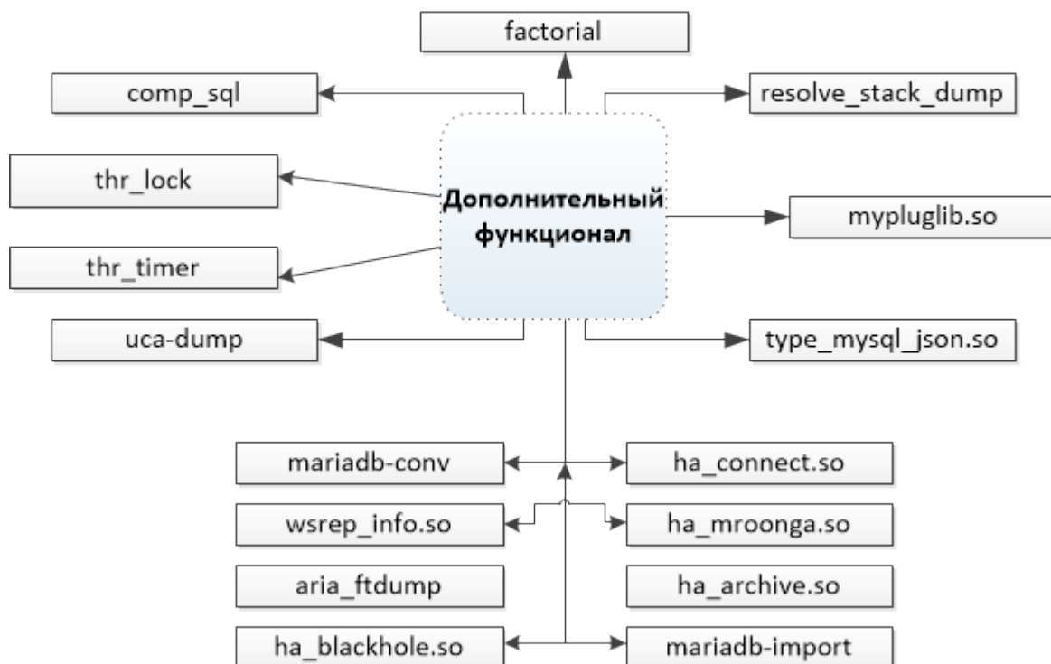
Рис.3 Структура подсистемы Расширения функциональности в СУБД «КАТРАПС»
